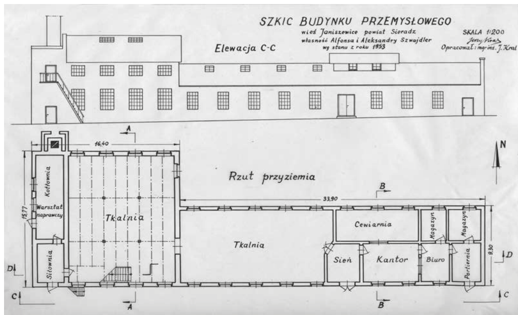
Ryc. 28. Plan fabryki A. Szwajdlera w Janiszewicach, przejętej przez SPCh „Argon” (1953)
